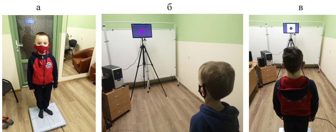
Рисунок 2. – Исследования на аппарате «Стабилан-01-2»
